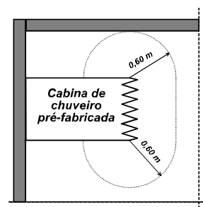
Fig. 701C — Cabina de chuveiro pré-fabricada (sem escala)
