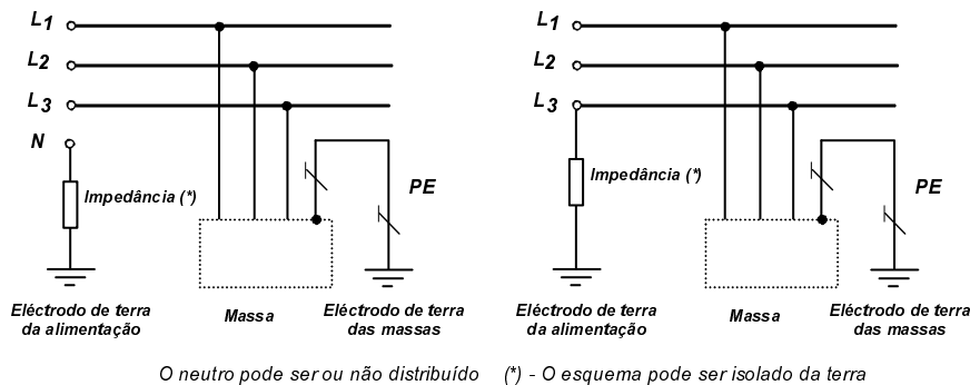
Fig. 31E — Esquema IT em corrente alternada (ac)
