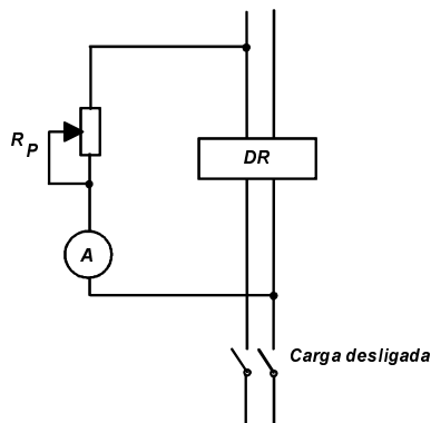
Figura B2 — Princípio de funcionamento do método 2
