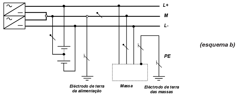
Figura 31 J — Esquema TT em corrente contínua (dc)
