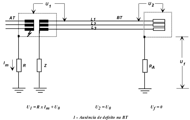
Fig. 44E — Esquema IT, exemplo «b»
