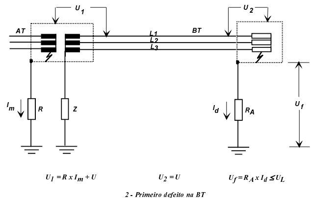
Fig. 44F — Esquema IT, exemplo «c1»
