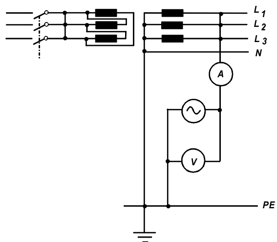
Figura D2 — Método da alimentação separada
