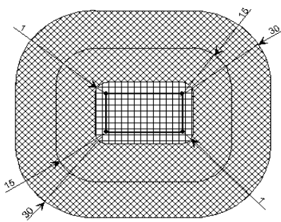
Fig. 801C — Zonas 1 (perigosa) e 2 (semi-perigosa) em reservatórios de gases sob pressão de densidade superior a 0,9, de altura não superior a 7,5 m e de capacidade superior a 200 m 3 .
