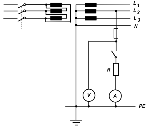
Figura D1 — Método das quedas de tensão
