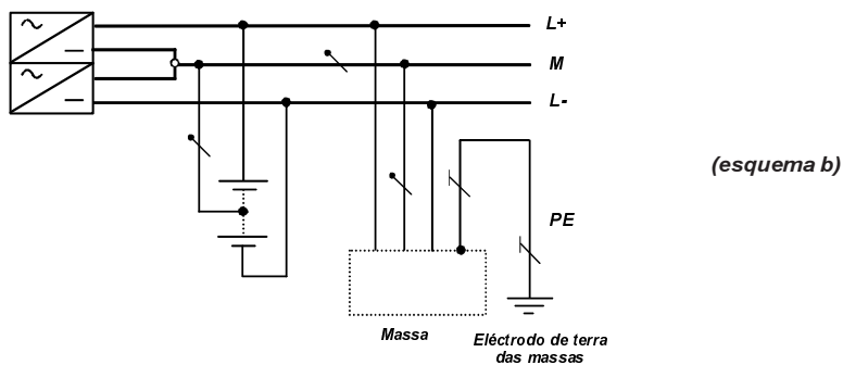
Figura 31 K — Esquema IT em corrente contínua (dc)
