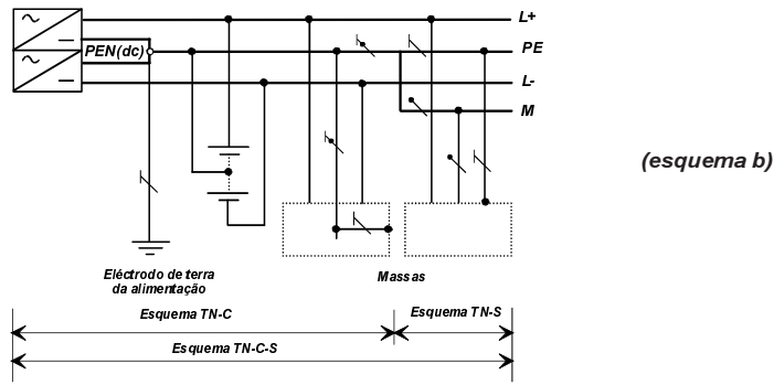
Fig. 31H — Esquema TN-C-S em corrente contínua (dc)
