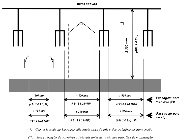
Fig. 48C — Passagens para serviço ou para manutenção nas instalações com partes activas dos dois lados, sem protecção.
