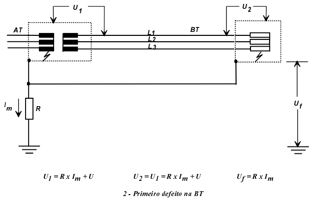
Figura 44K - Esquema IT, exemplo «e2»
