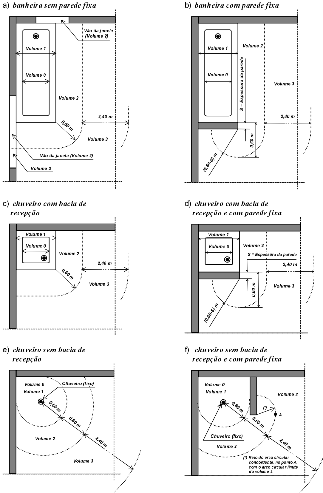
Fig. 701A — Exemplos de dimensões dos volumes em casas de banho (planta) (sem escala)
