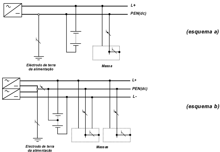
Fig. 31G — Esquema TN-C em corrente contínua (dc)
