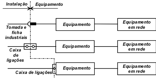
Fig. A1 — Fronteiras entre as instalações e os equipamentos
