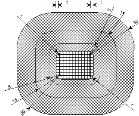
Fig. 801D — Zonas 1 (perigosa) e 2 (semi-perigosa) em reservatórios de gases sob pressão de densidade superior a 0,9, de altura superior a 7,5 m e de capacidade superior a 200 m 3 .
