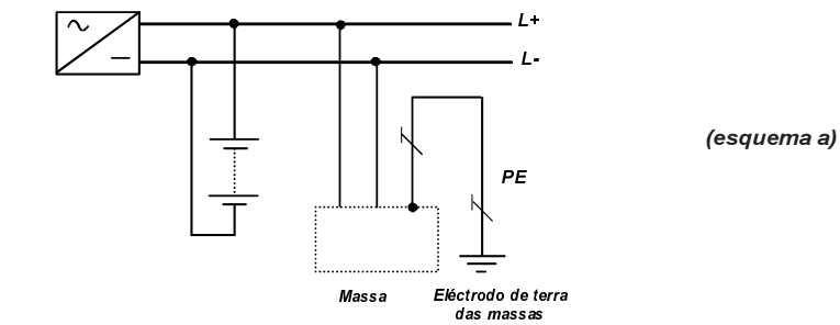
Figura 31 J — Esquema TT em corrente contínua (dc)
