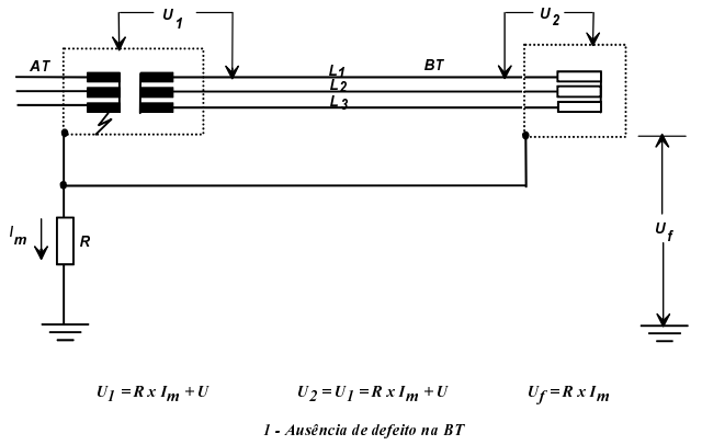
Figura 44J - Esquema IT, exemplo «e1»
