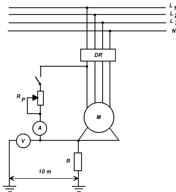
Figura B3 — Princípio de funcionamento do método 3
