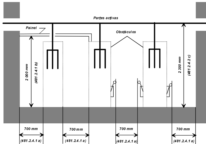
Fig. 48A — Passagem para serviço ou para manutenção nas instalações com protecção por meio de obstáculos
