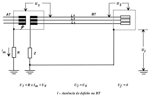
Fig. 44G — Esquema IT, exemplo «c2»
