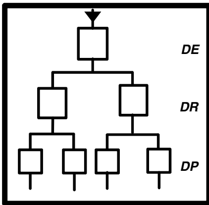
Figura 47GT — Quadro de distribuição da classe II, com invólucro metálico
