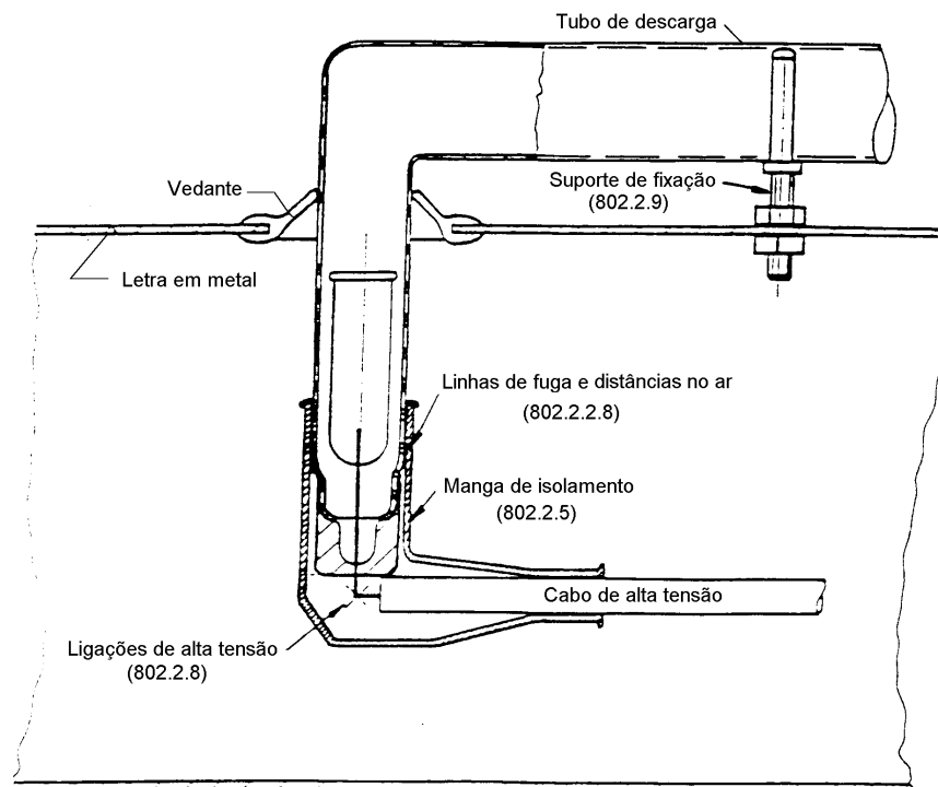
Fig. 3 — Exemplo de uma ligação de alta tensão com um electrodo a atravessar um painel metálico.
